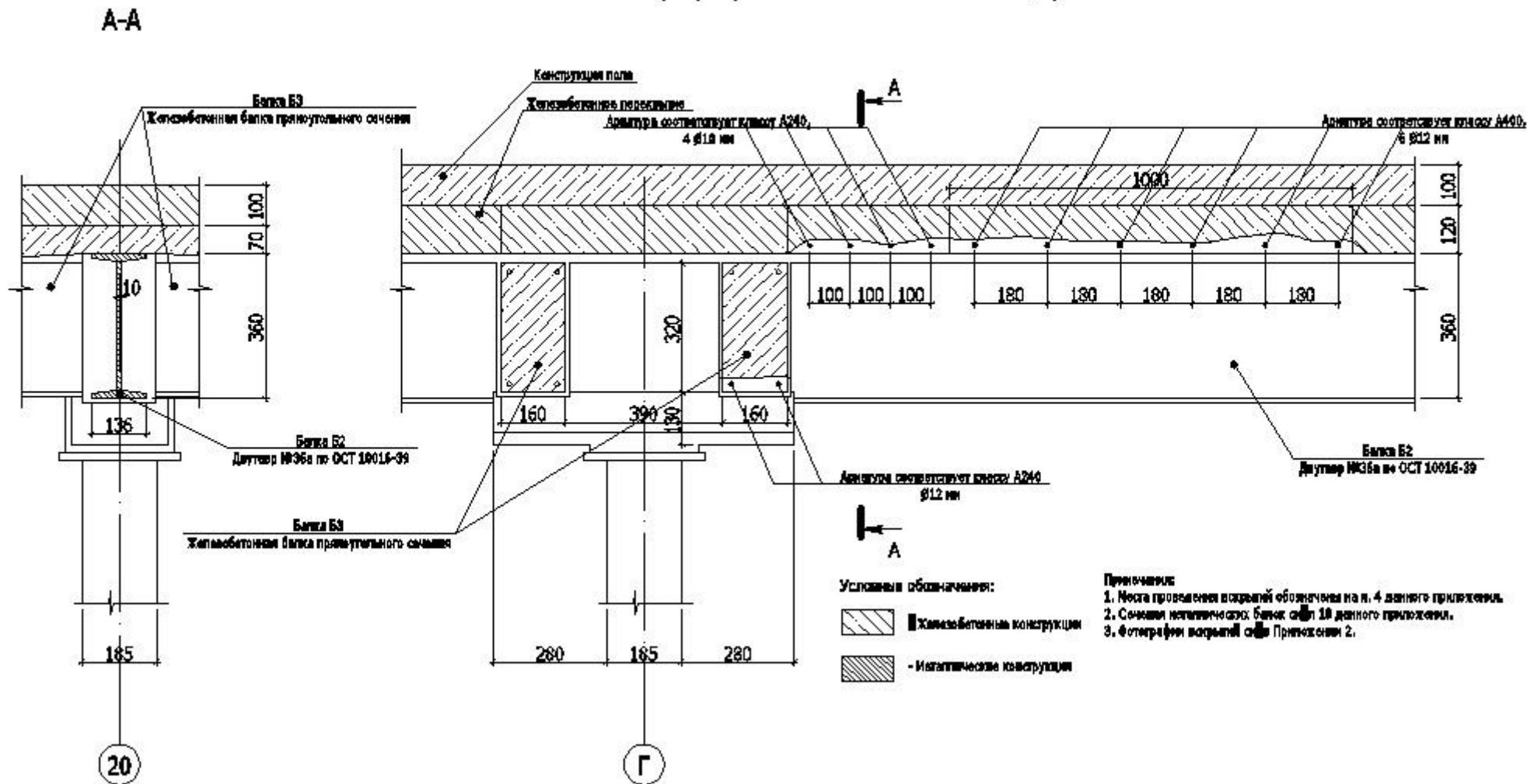
Вскрытие № 11. М 1:10. (Перекрытие 3-го этажа в осях 20/Г)
